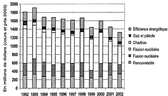
Budgets de la recherche en matière d'énergie des pays européens membres de l'AIE 1992-2002 (Allemagne, Autriche, Belgique, Danemark, Espagne, Finlande, France, Grande-Bretagne, Grèce, Hongrie, Irlande, Italie, Luxembourg, Pays-Bas, Portugal, Suisse, Tchéquie)
